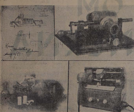
Bilderna visa översikt Edisons första skiss till fonografen och den första exemplaret till ett gramfon. De två andra bilderna visa Edison i arbete och den senaste ljudregistreringsapparaten Electric.
