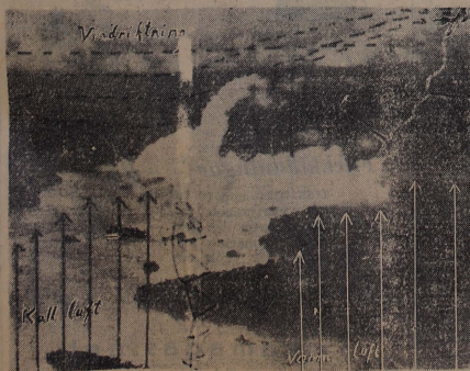
En bild som belyser segelflygning över ett kuperat landskap.
