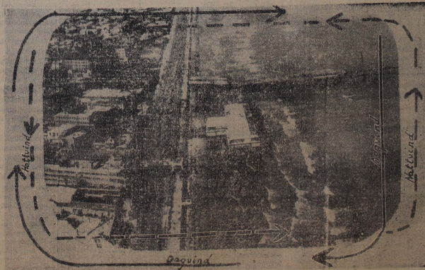
Växelverkan mellan luftströmmarna om dagen och natten i en kusttrakt.
