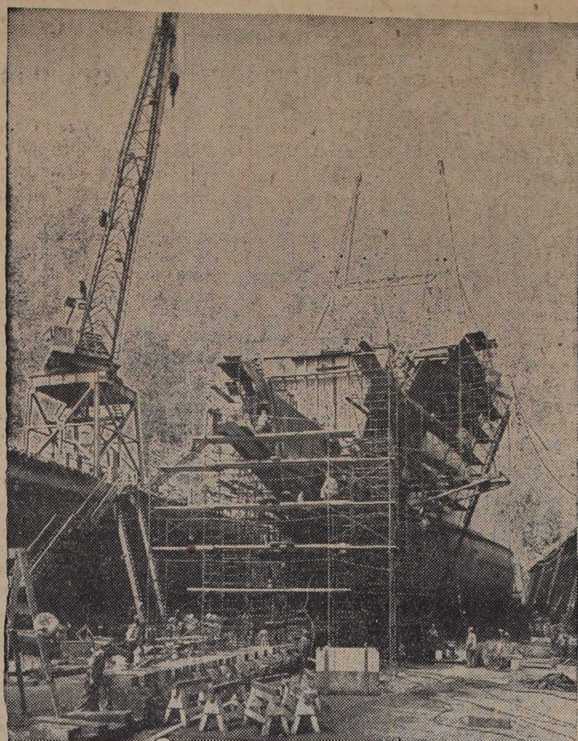
Reparationsarbetet med Amerikaliniens Stockholm fortskrider i rask takt. Hela frampartiet var skadat och delvis borta när fartyget lades i torrdocka. Arbetet med plåtarna under vattenlinjen är nu klart och man arbetar med överdelen. Innan fartyget är helt klart återstår sedan inredningsarbeten i fören samt komplettering av utrustningen såsom nya ankare och kätting.
