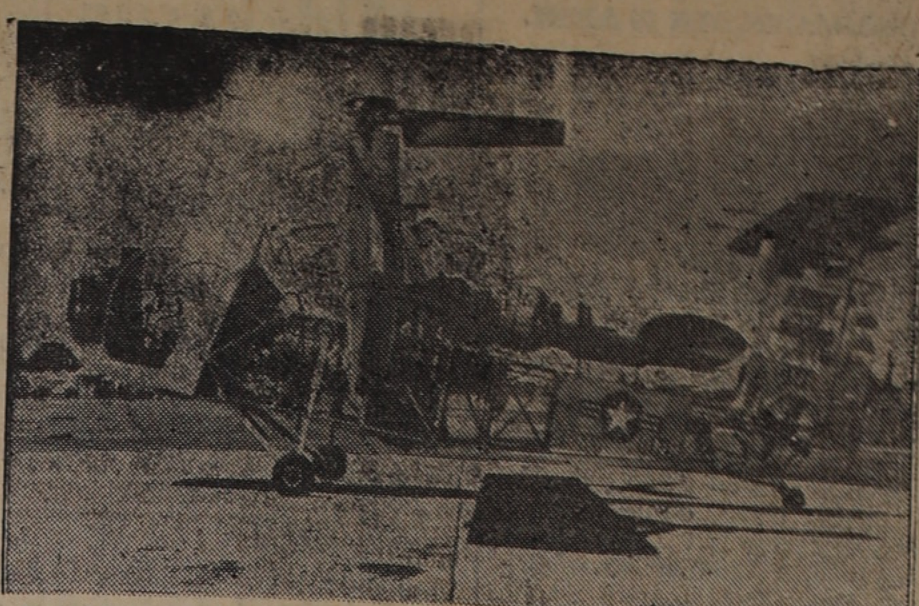
Det här amerikanska planet är det första i sitt slag och kan med en enkel manöver förvandlas till helikopter eller till en helt vanlig maskin för planflykt. På bilden har de två motorerna och vingarna flöjats vägrätt, varvid planet startar och landar som en helikopter. För vanlig flygning ställs bara vingarna och motorerna horisontellt.
