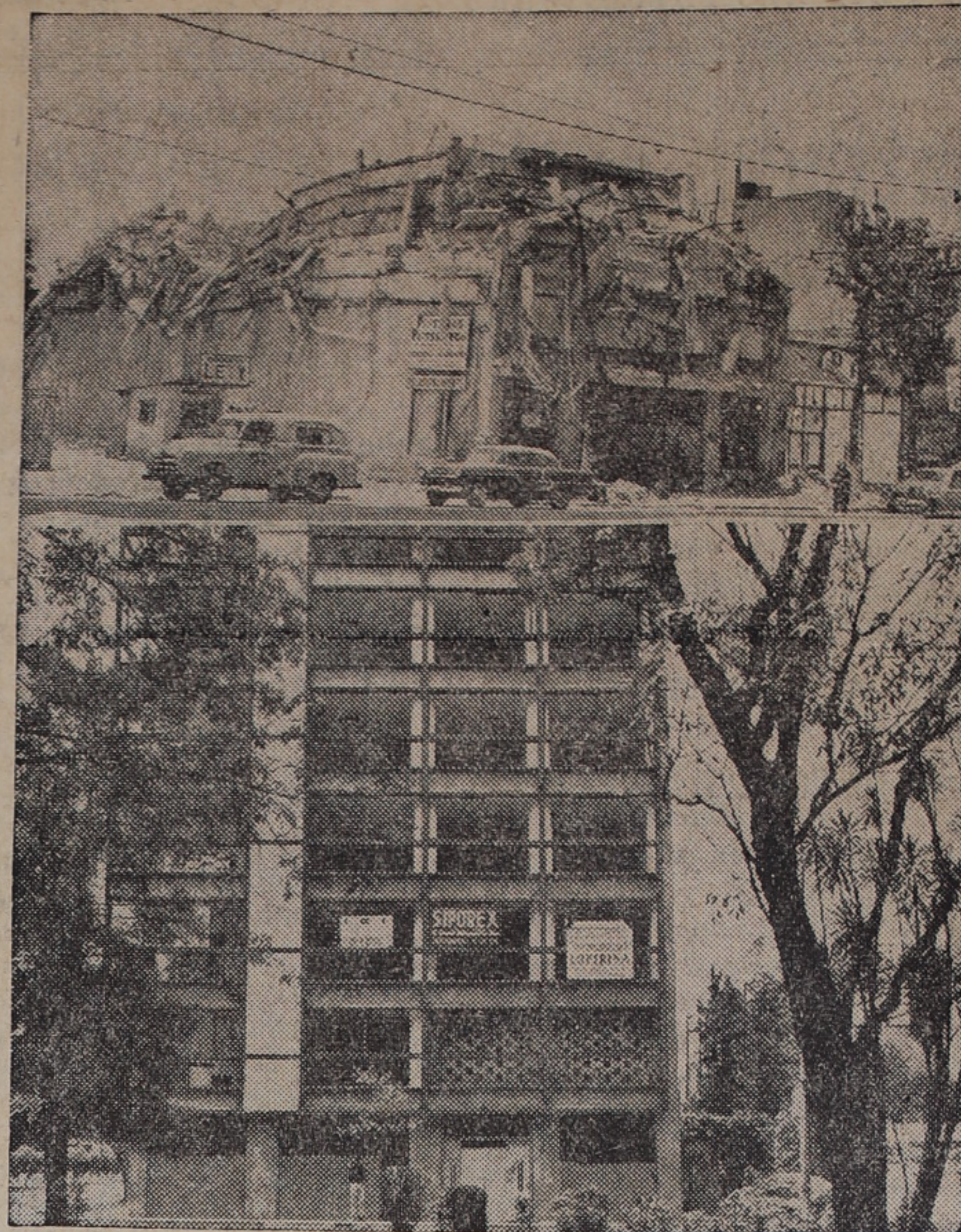
En typisk bild från Mexico City just nu. Överst ett vanligt sexvåningarshus som jordbävningen tryckt samman. Observera bjälklagen ovanpå varandra. — Under ett hus av Siporex, som inte ens fått en spricka.
