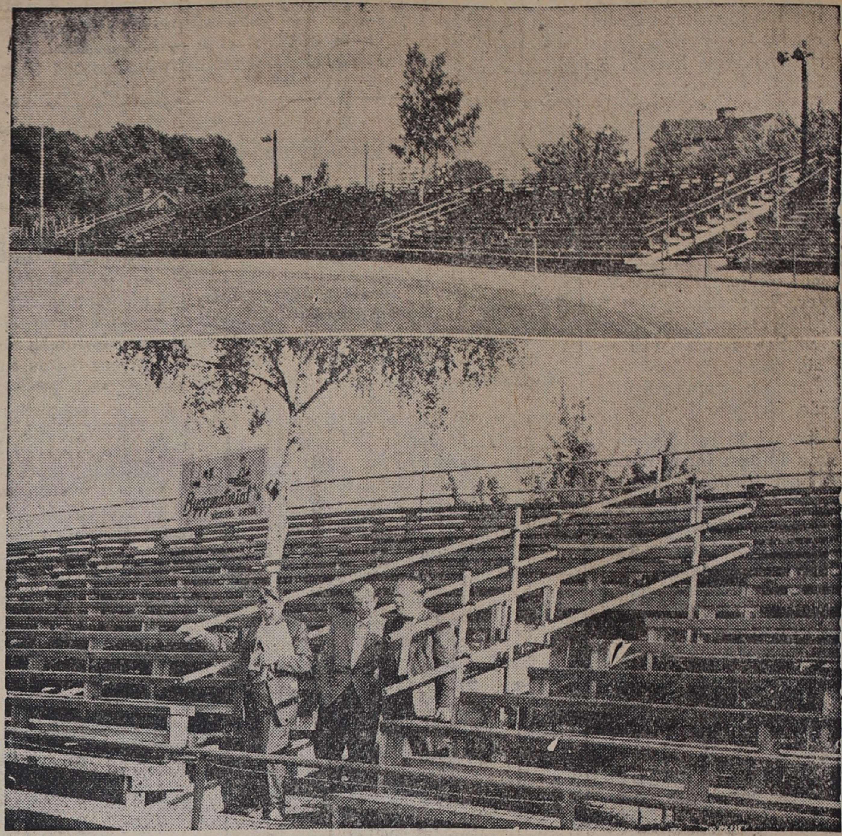
"Västerås-läktarna" håller på att erövra de svenska idrottsarenor. Konstruktionen baserar sig på rörkopplingar och monteringen kan ske på rekordtid. På övre bilden del av nya sittplatsläktaren på Aros-vallen i Västerås med plats för 2.700 personer. På undre bilden informerar disponent Ake Hultström, Västerås Byggnadsmaterial (i mitten) om de revolutionerande läktarkonstruktionerna. Här flankeras han av två idrottsplaterepresentanter, N A Bergman och Hubert Bergvall från Kristinehamn under den kongress idrottsplatsernas riksförbund i dagarna hållit i Västerås.
