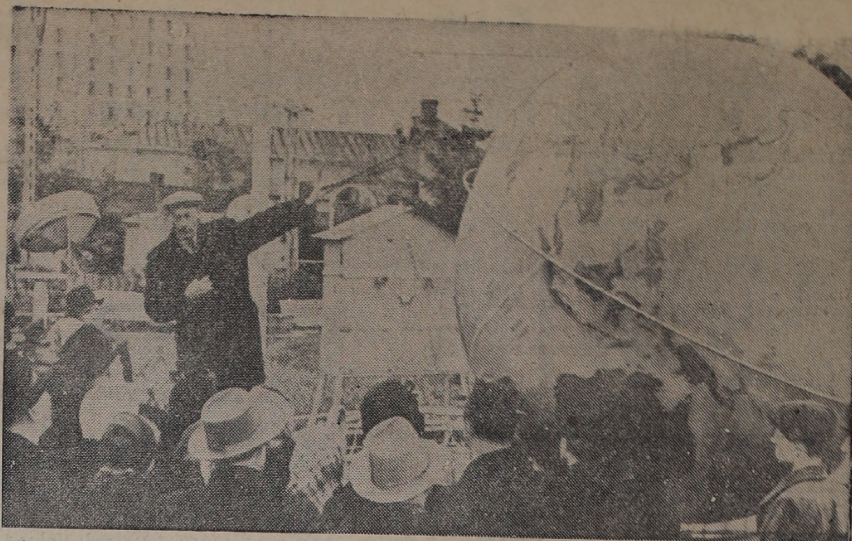
På Astronomitorget i Moskva framför ett av Moskas observatorier håller R. Zvetov en föreläsning för allmänheten om hur den ryska satelliten kretsar kring jorden. Man kan se satellitens bana markerad som en ring runt den väldiga jordgloben.
