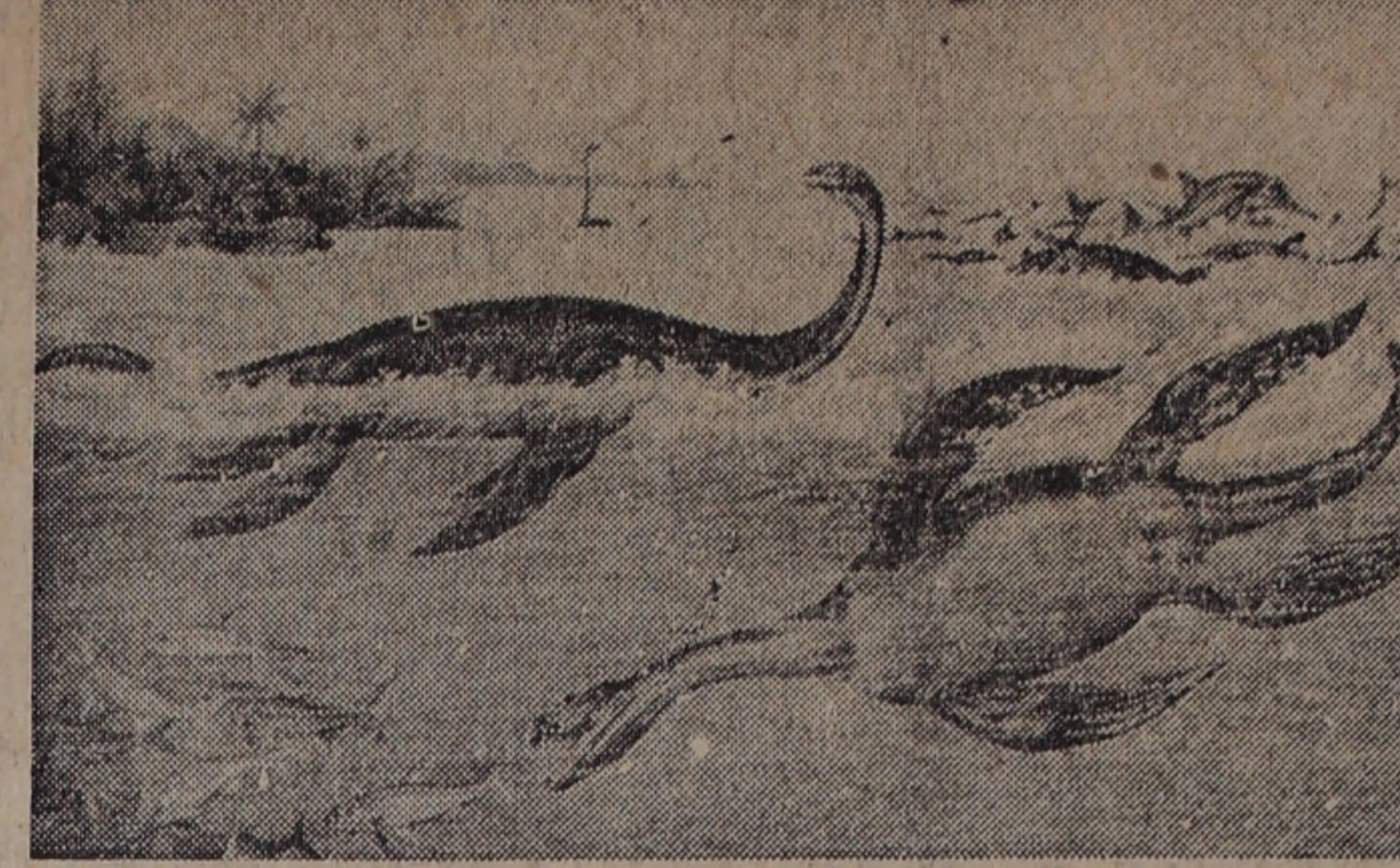
Det var i urtidens ljumma hav som livet uppstod och utvecklades. Här är havsdölar från juraperioden.
