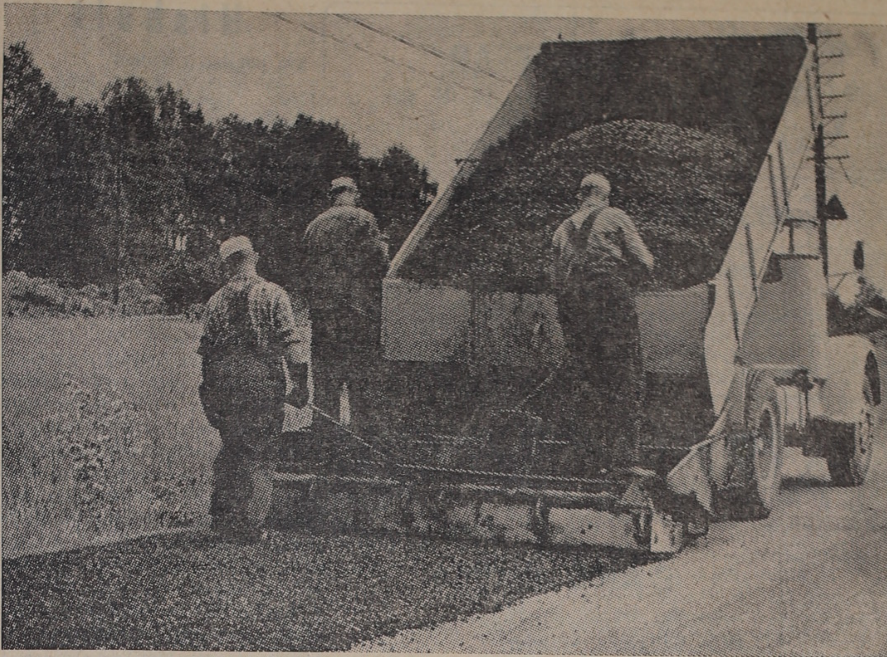
MEÐ ETT ENKELT aggregat kopplat till "grusbilen" lägger man ut olje-gruset på vägen. Det är inga tjocka lager man behöver lägga på. I regel räcker det med ett fyra centimeter tjockt ytskikt.
