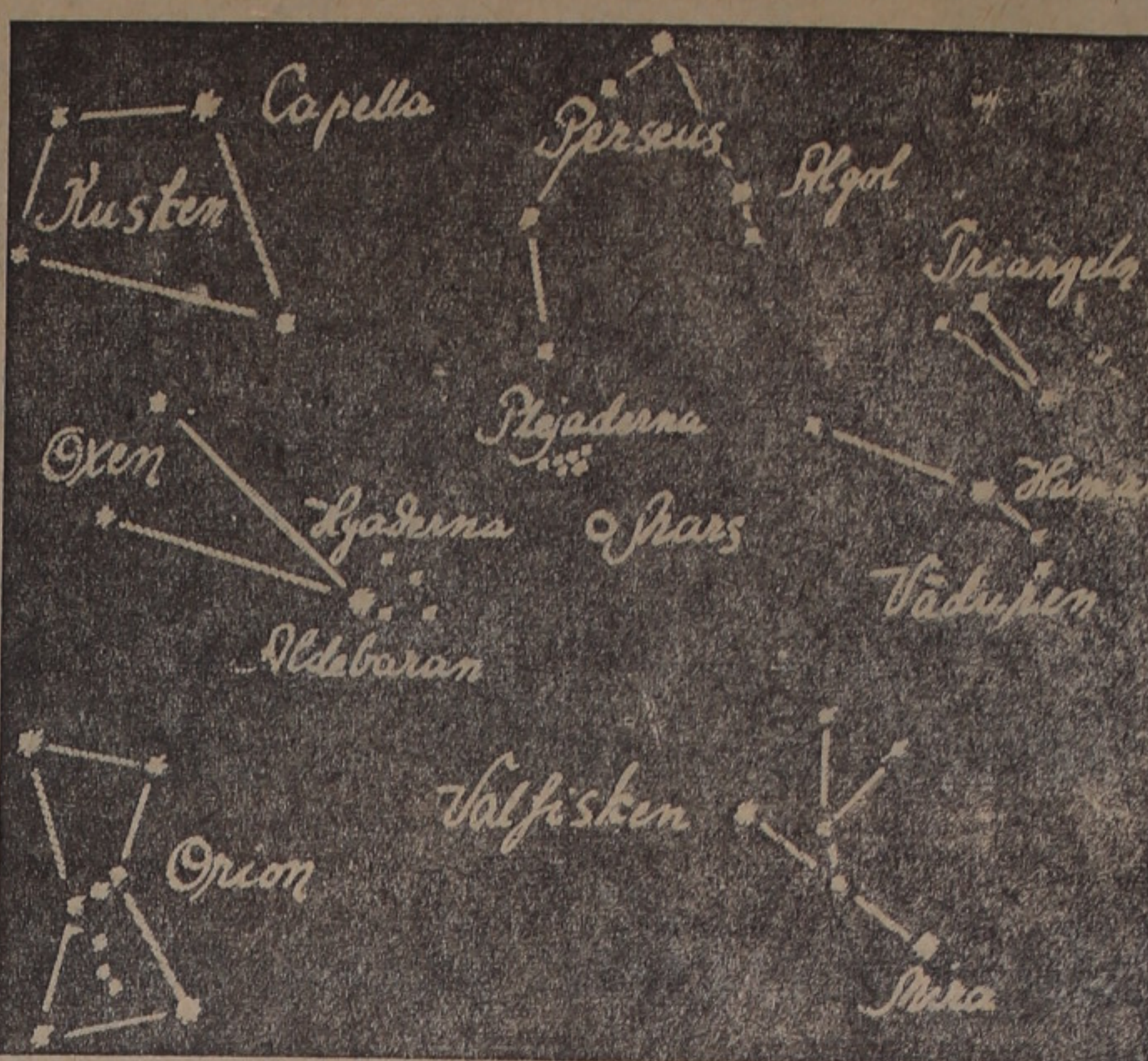
Några av de klarast lysande stjärnkonstellationerna på februarihimlen.
