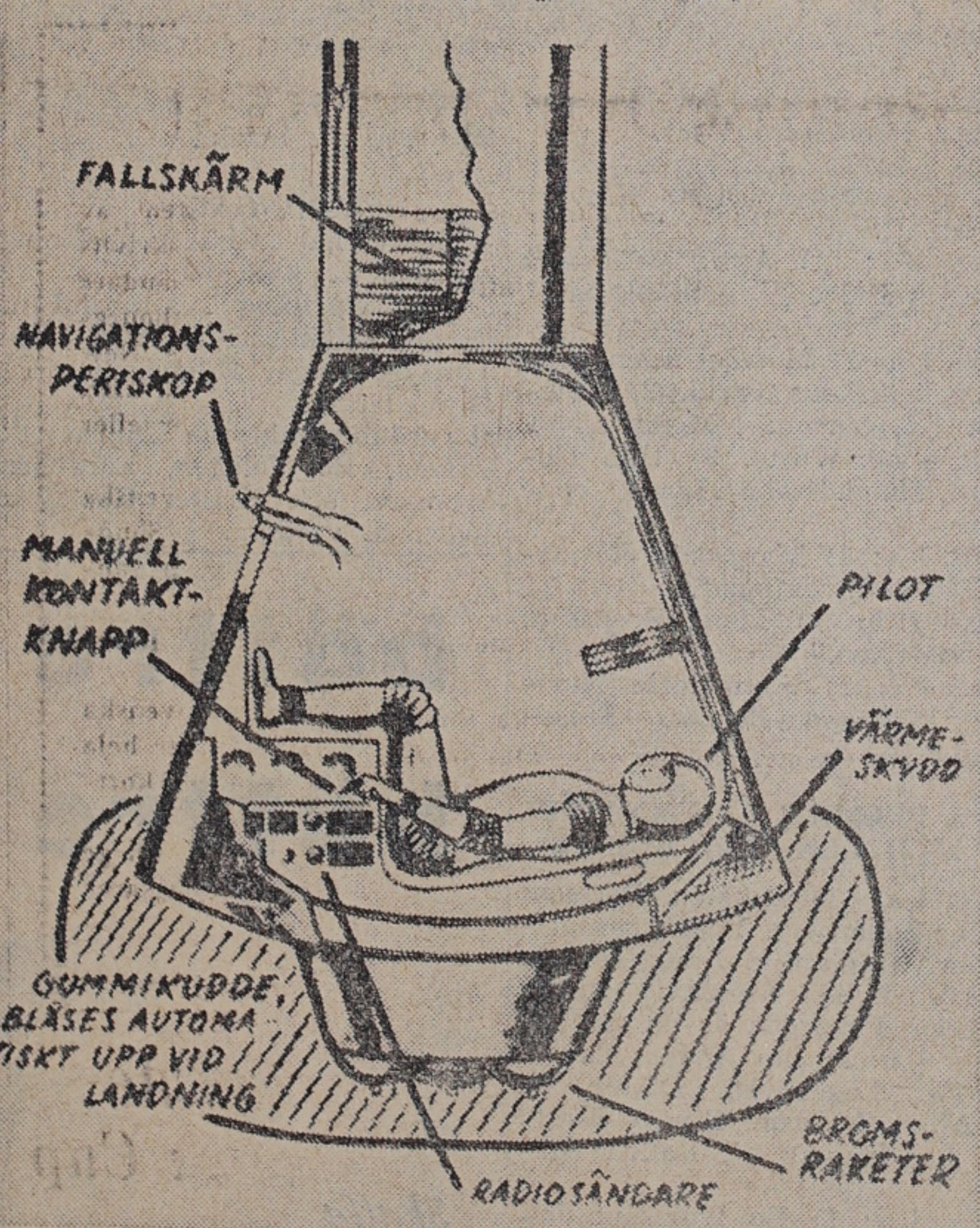
En teckning av den rymdkon, där rymdmannen skall ligga fastspänd.
