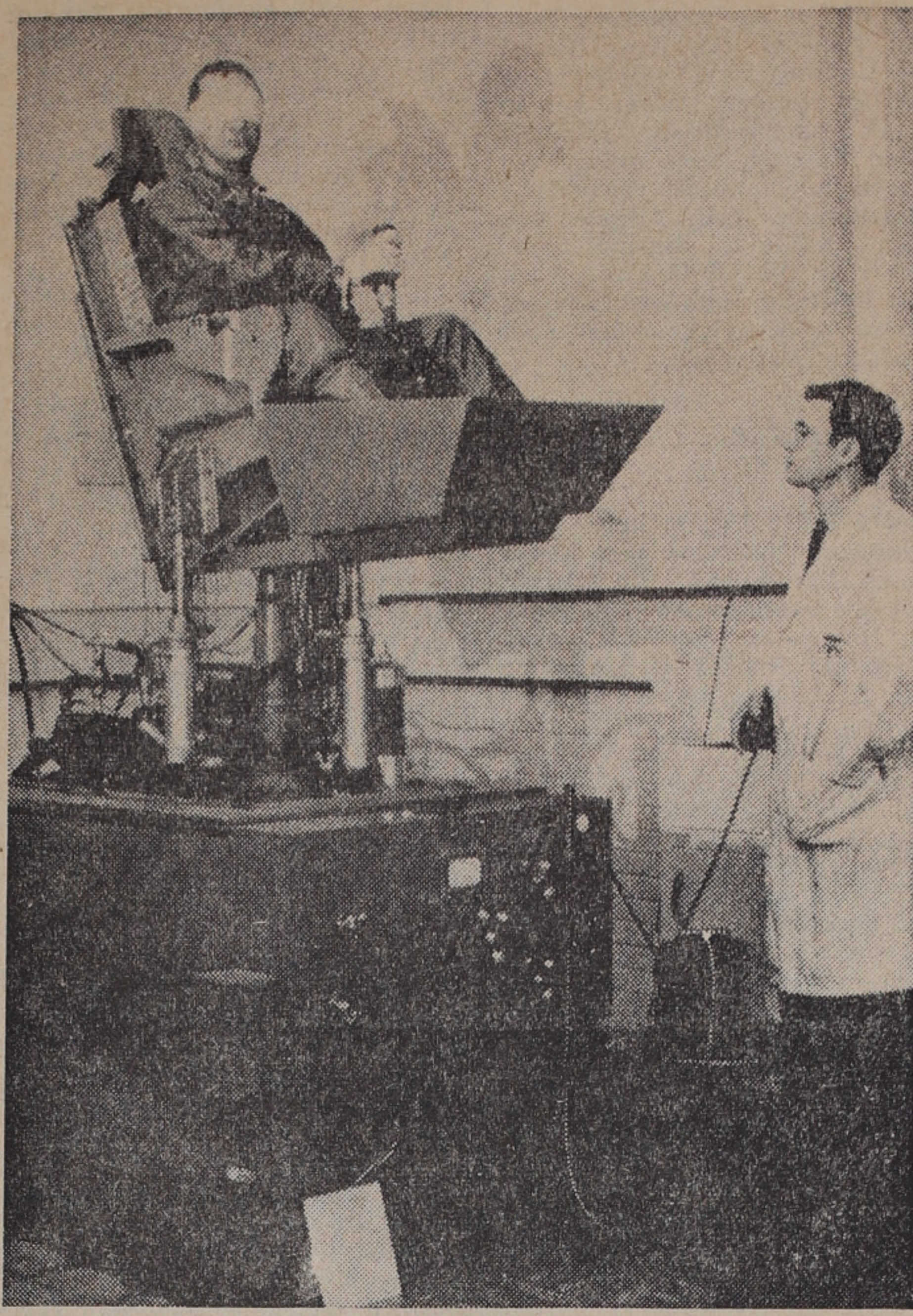
En av de sju, flygkapten Grissom, genomgår balanstest i en stol som roterar på två axlar samtidigt. Med hjälp av en styrspak skall han försöka hålla stolen i horisontalläge.
