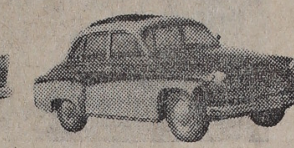
WARTBURG DE LUXE 5 pers, 4 dörrar, 3 cyl, 40 hk DIN, skatt 166, oms 1.100, pris 9.700 kr.
