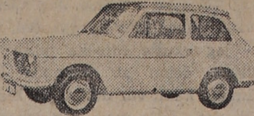
AUSTIN A 40 4 pers, 2 dörrar, 4 cyl, 38 hk SAE, skatt 110, oms 920, pris 7.695 kr.
