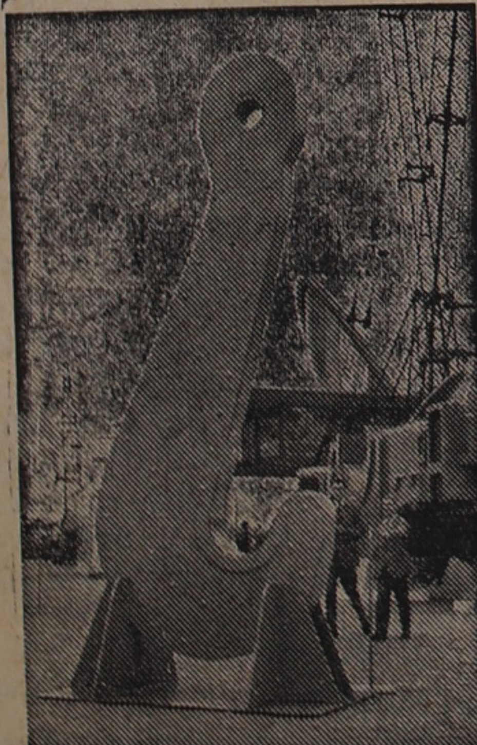
En krankrok av mer ovanliga dimensioner än den här, som framställdes i Tyskland i lamellkonstruktion. Kroken mäter 7,7 m och väger 8.580 kg, men så kan den också ta en last på 174 ton. Den enorma kroken är avsedd för ett stälverk i Argentina.
