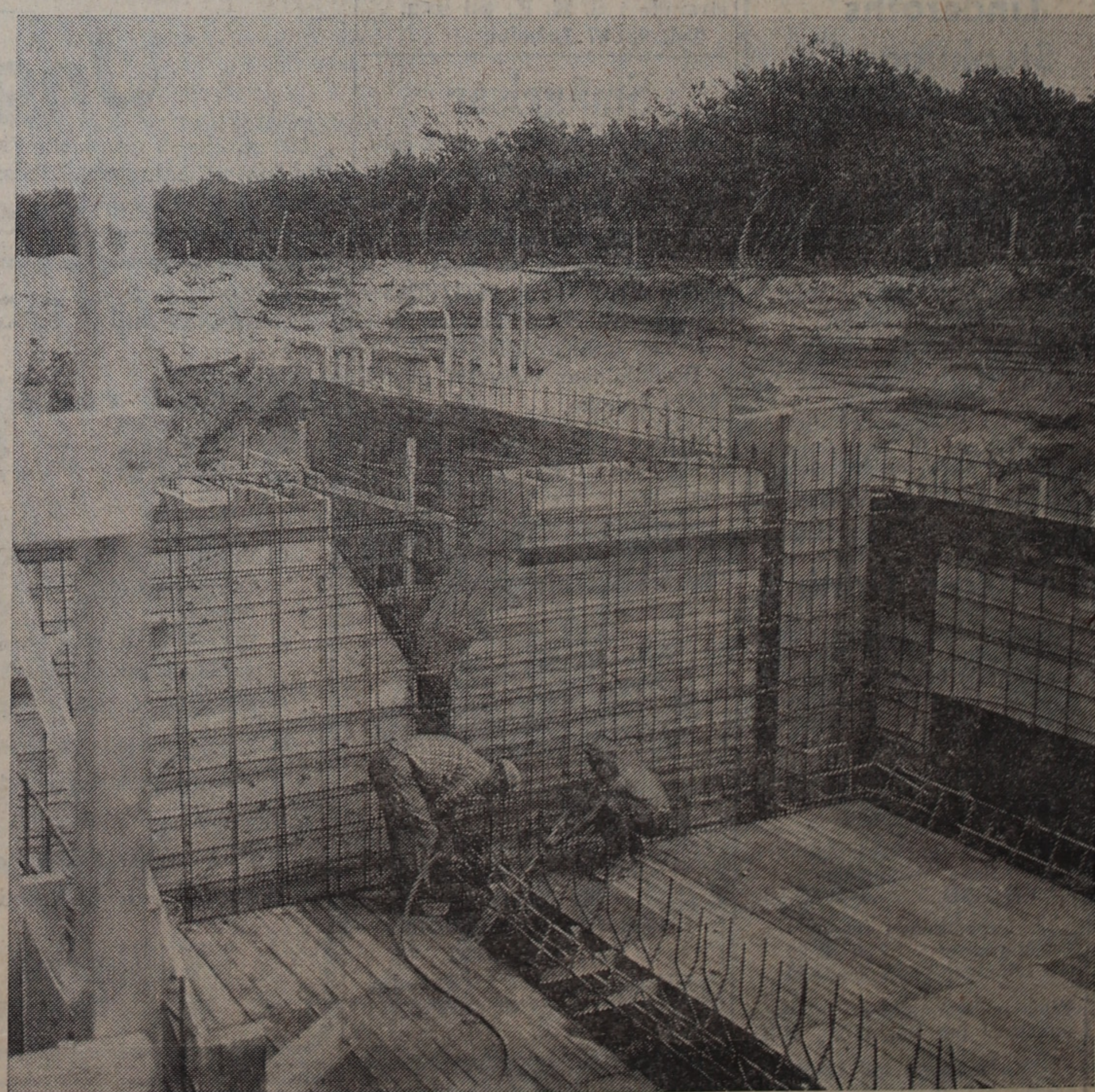
Den 90 meter långa och 5 meter djupa reningsbassängen i Skummeslövsstrand börjar ta form
