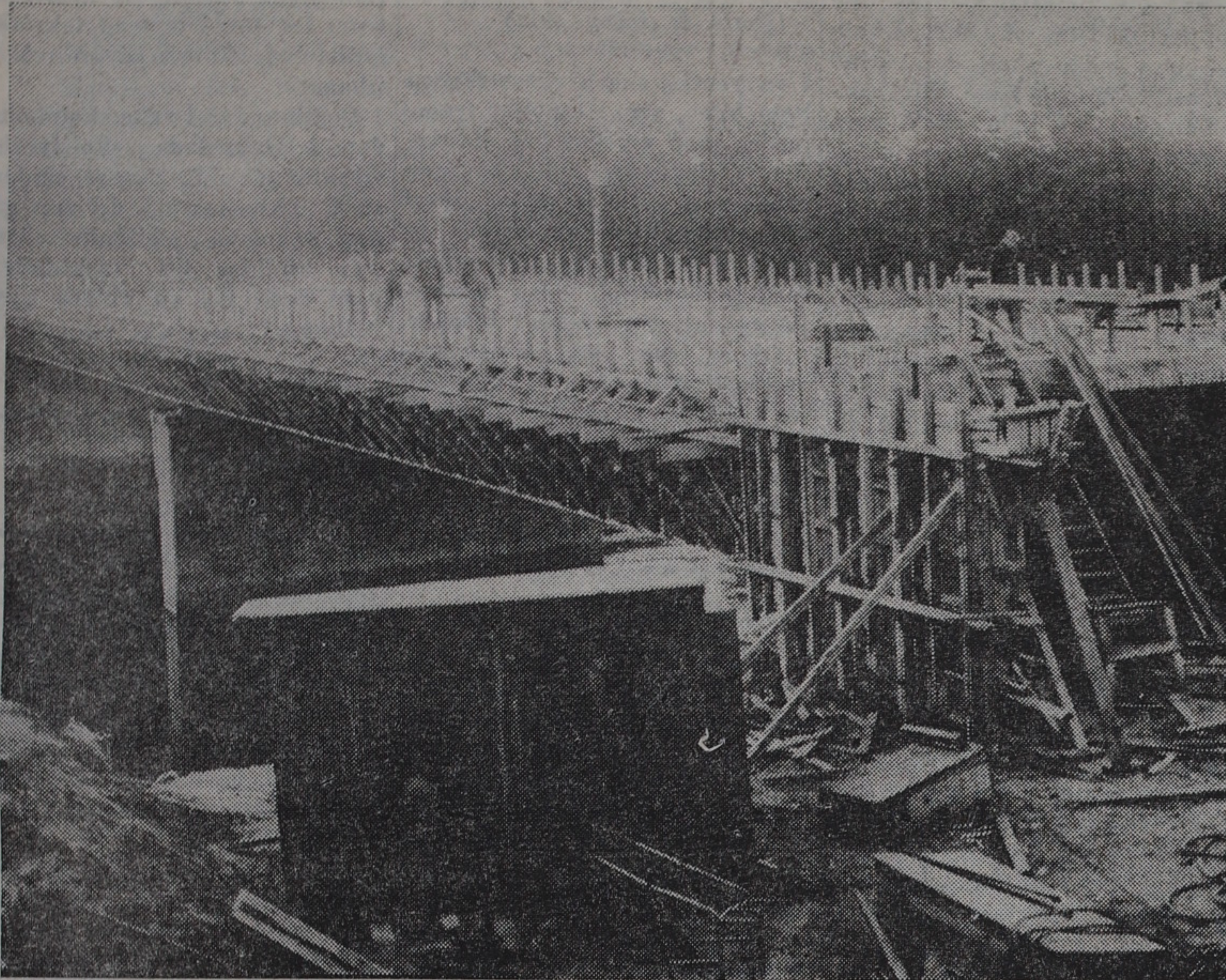
Snickarna i fullt arbete med formar för gjutningen av bron över Lagan
