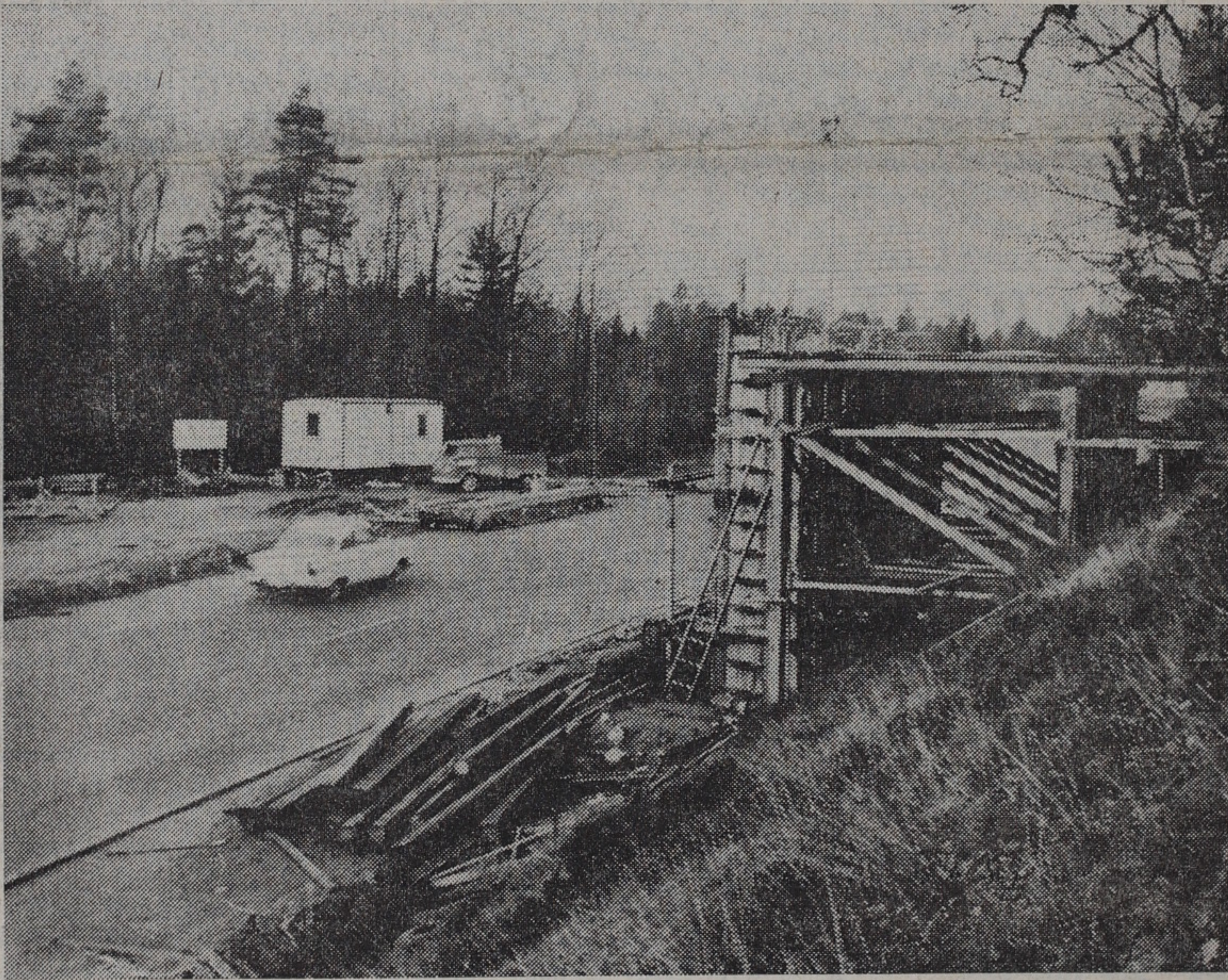
Den blivande viaduktens grundgjutning sedd från norra sidan av Hässleholmsvägen.
