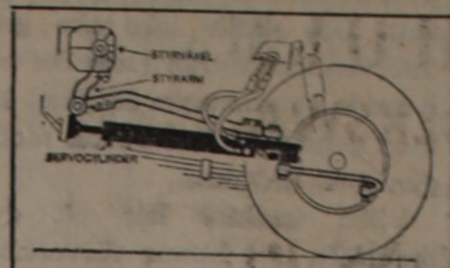
Servostyrning — nyhet som gör Raske Tiptop ännu mer lättmanövrerad.
