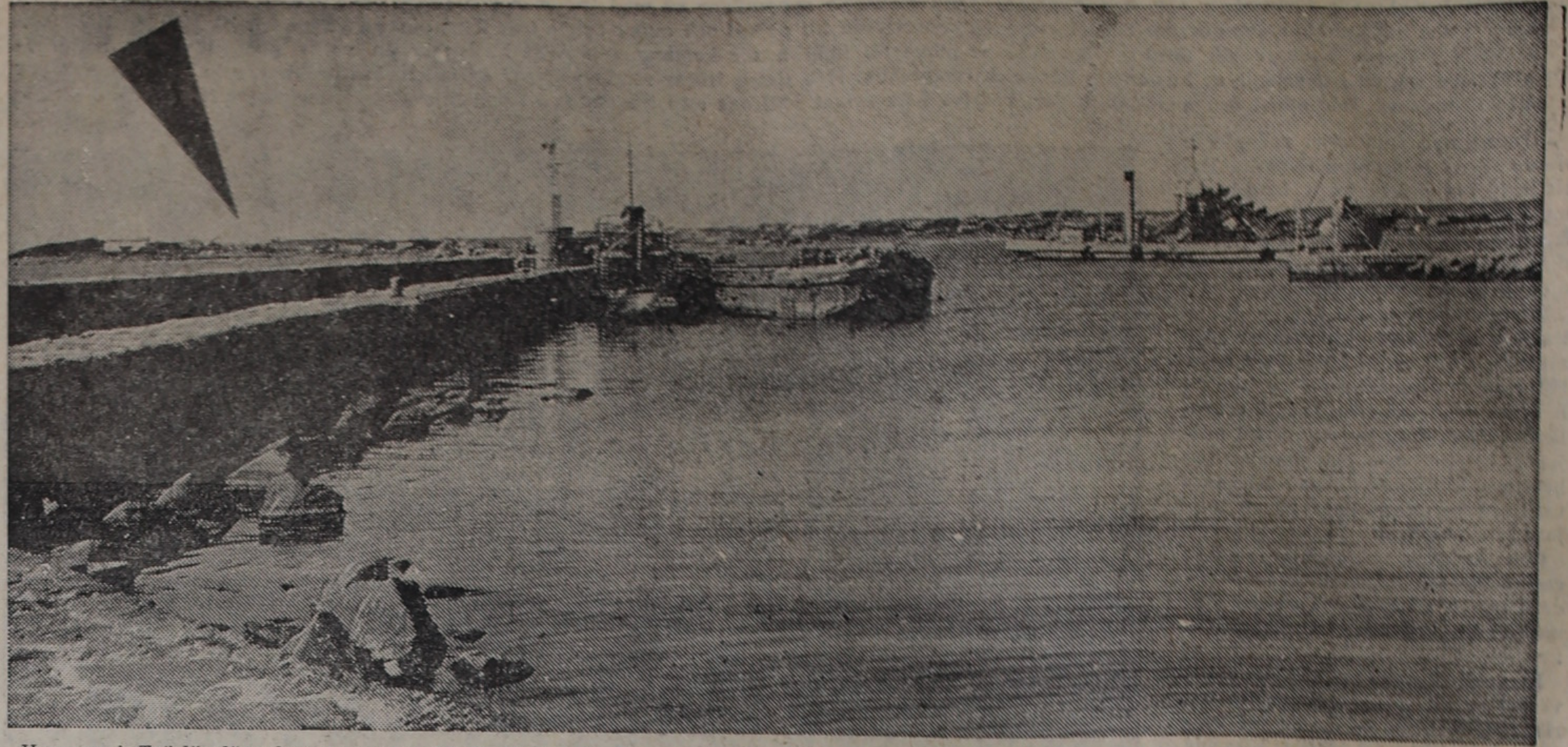
Hamnen i Träslövsläge kommer att radikalt förändras. Det gamla hamninloppet, mellan mudderverket och prämen pluggas igen och ett nytt inlopp tas upp genom att man helt enkelt skär igenom den gamla vägbrytaren (vid pilen).
