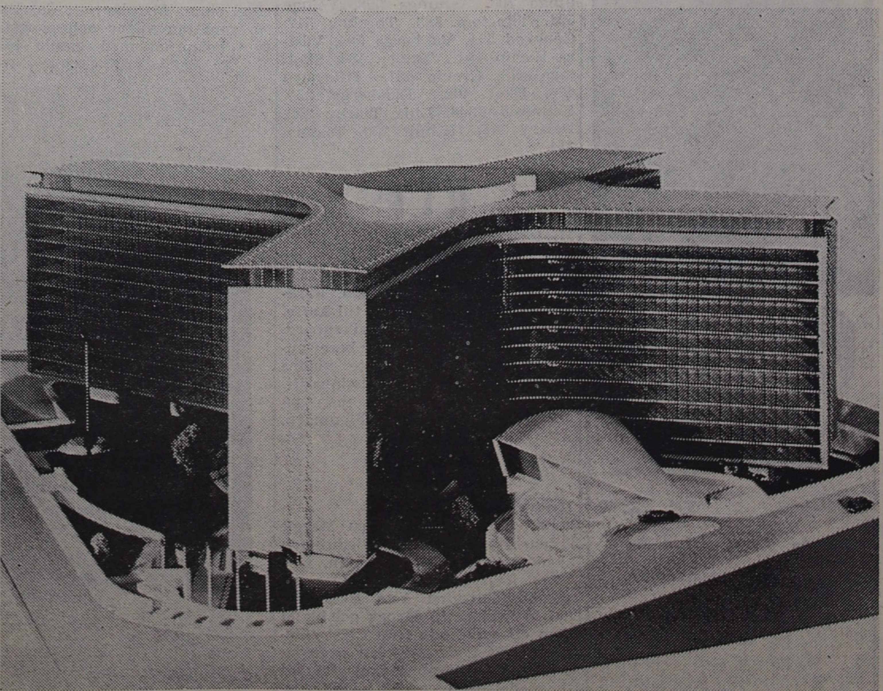
Mitt i hjärtat av Bryssel reser sig det höghus i vilket hela EECs organisation ska inrymmas. Den första delen av byggnaden kommer att tas i bruk 1966. Tre år senare ska höghuskomplexet tillsammans med fyra flyglar härberga 5.500 europatjänstemän. En egen underjordisk järnvägsstation kommer att förbinda lokalerna med Europas huvudstäder.
