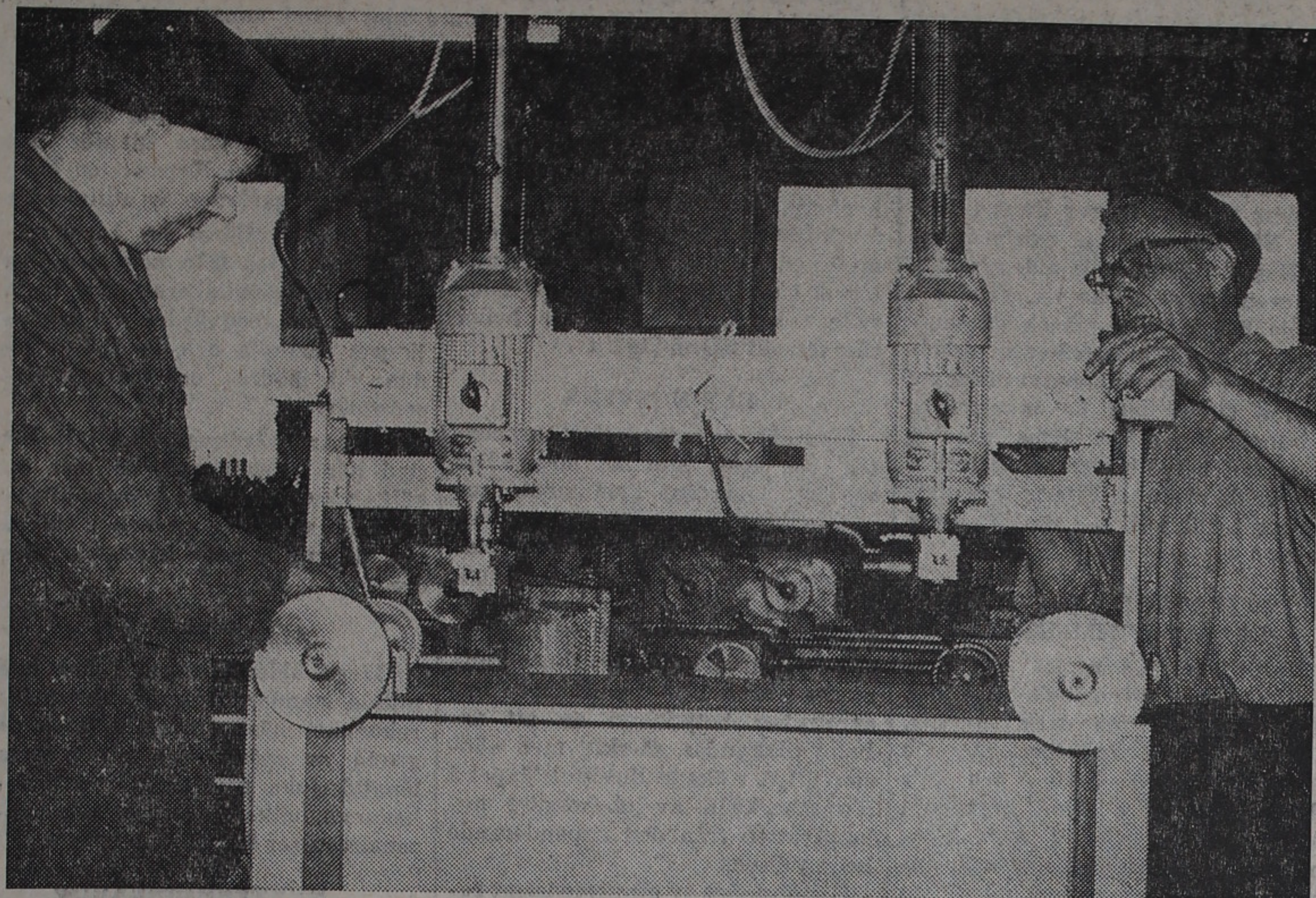
På bilden syns Olle Bruno och Stig Larsson vid en flerspindlig tappmaskin med el. och luft. Maskinen är nu i det närmaste färdig och skall tagas i bruk efter semestern vid en av ortens snickerifabriker.
