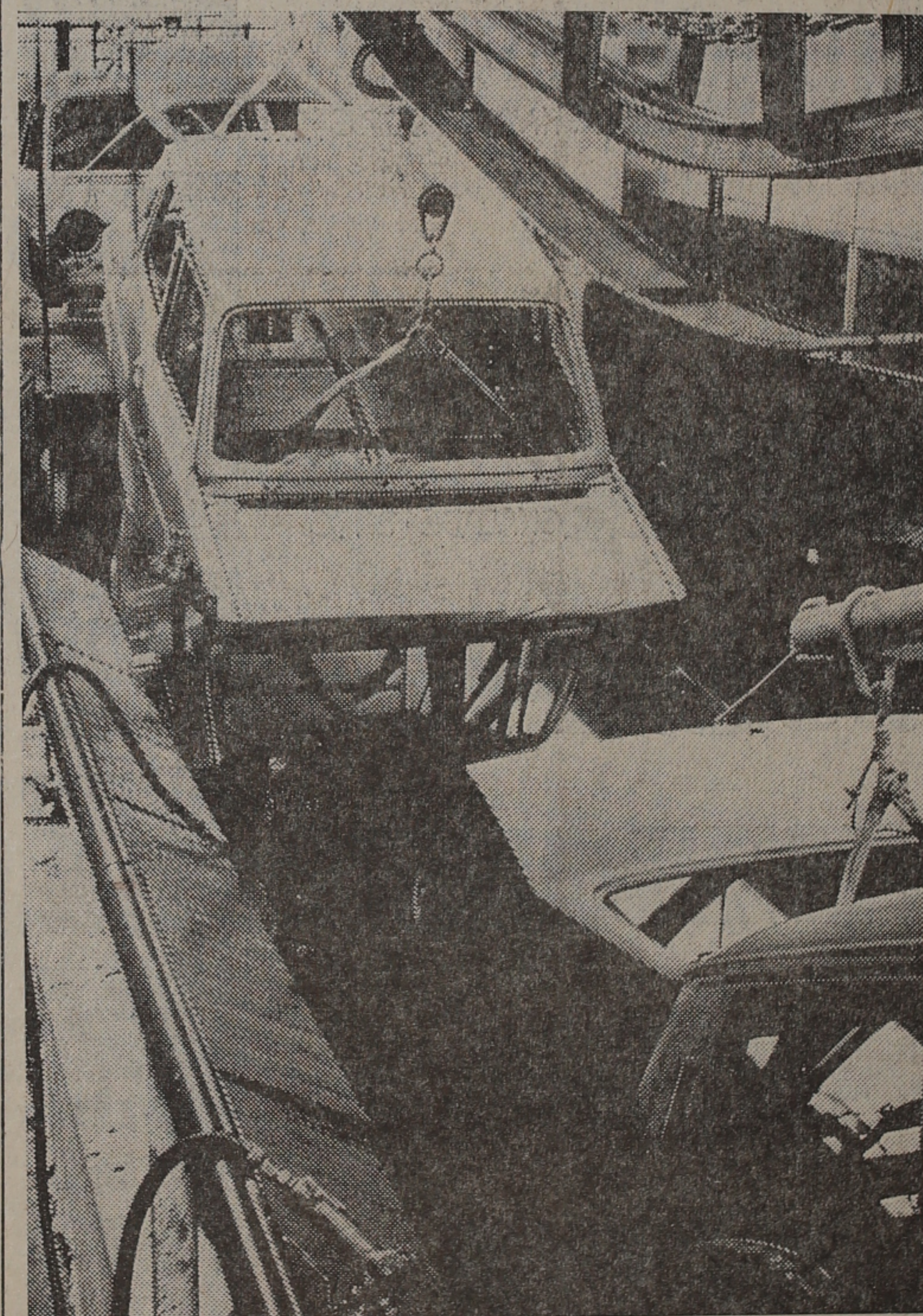
Karosser till Simca 1100 på väg genom vinylbadet.
