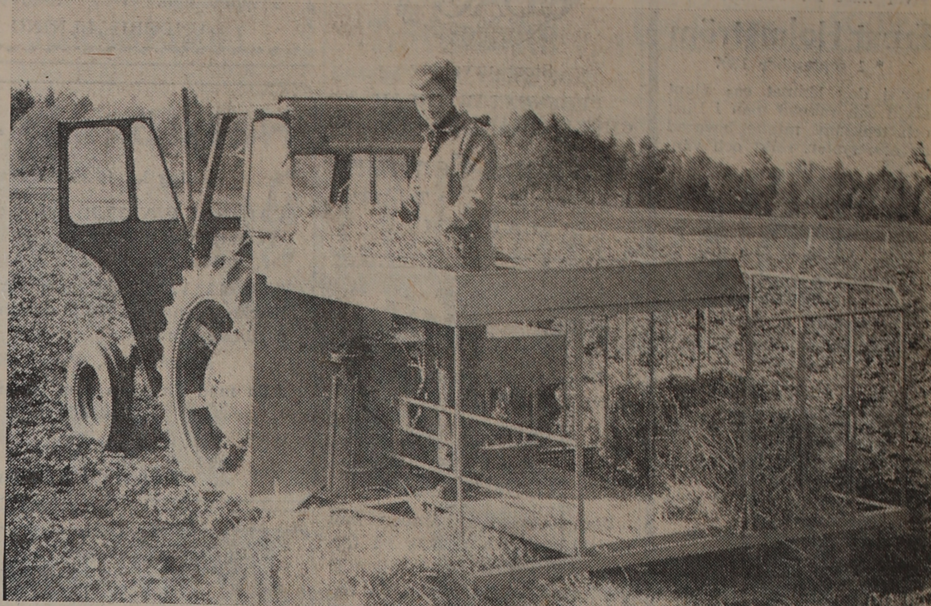
En av de maskiner som kommit fram på senare år är denna halmstridare, som lägger halm mellan jordgubbsraderna för att förhindra nedsmutsning av bären.
