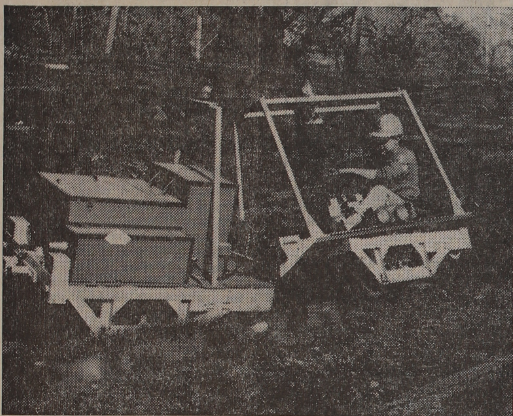
Nelsons fordon för svår terräng heter den tvådelade kärran på bilden, som rullar på Goodyears breda lågtrycksdäck med utpåkigande drivmat. Det klarar stigningar på 50 procent. Vikten är 1.050 kg och marktrycket ca 0,1 kg/cm 2 . Fordonet har en dragkraft på drygt 500 kg i lös sand och ca 830 kg på asfalt eller betong. Vändradien är 2,5 m.
