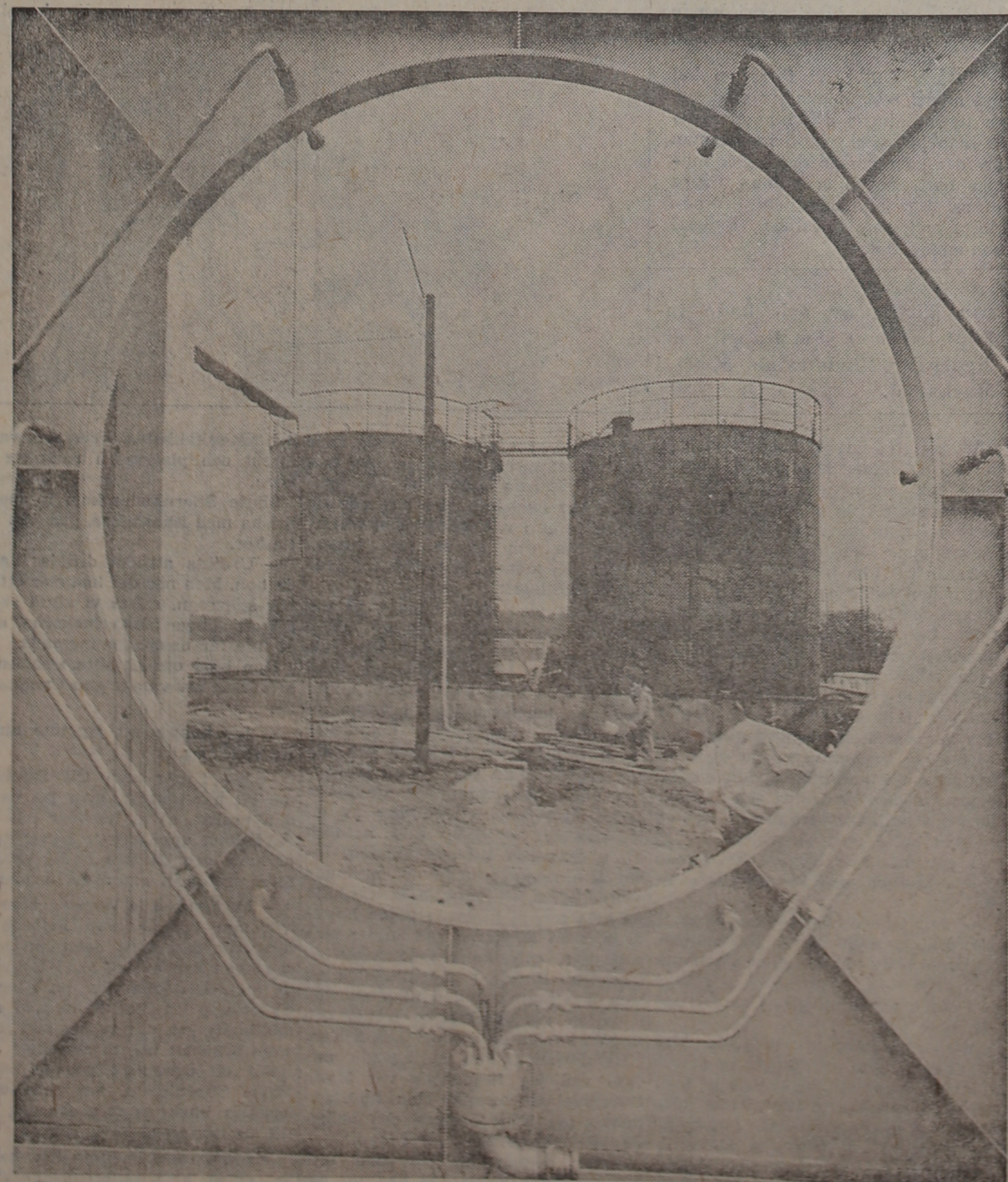
Cisternerna vid det blivande spetskraftverket i Falkenberg. Dessa rymmer 250 kbm vardera och skall tjäna som bränsleförråd. Bilden tagen genom en av turbinstationens vägar av i. Fotoarjen Larsson.
