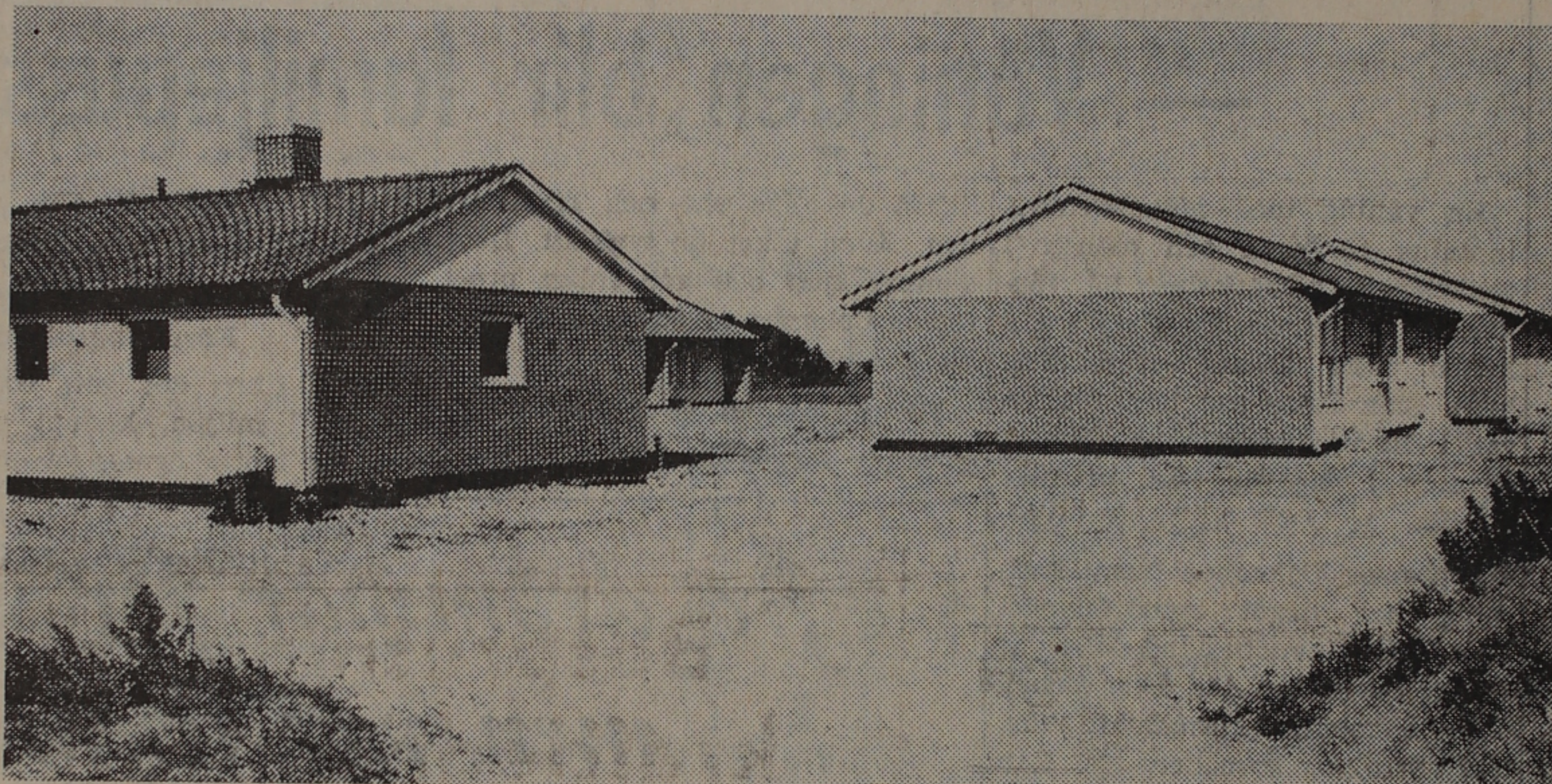
Pensionärsbostäderna i Skottorp. Byggnaden till vänster inrymmer gillesstuga, panncentral, tvättstuga och pentry.
