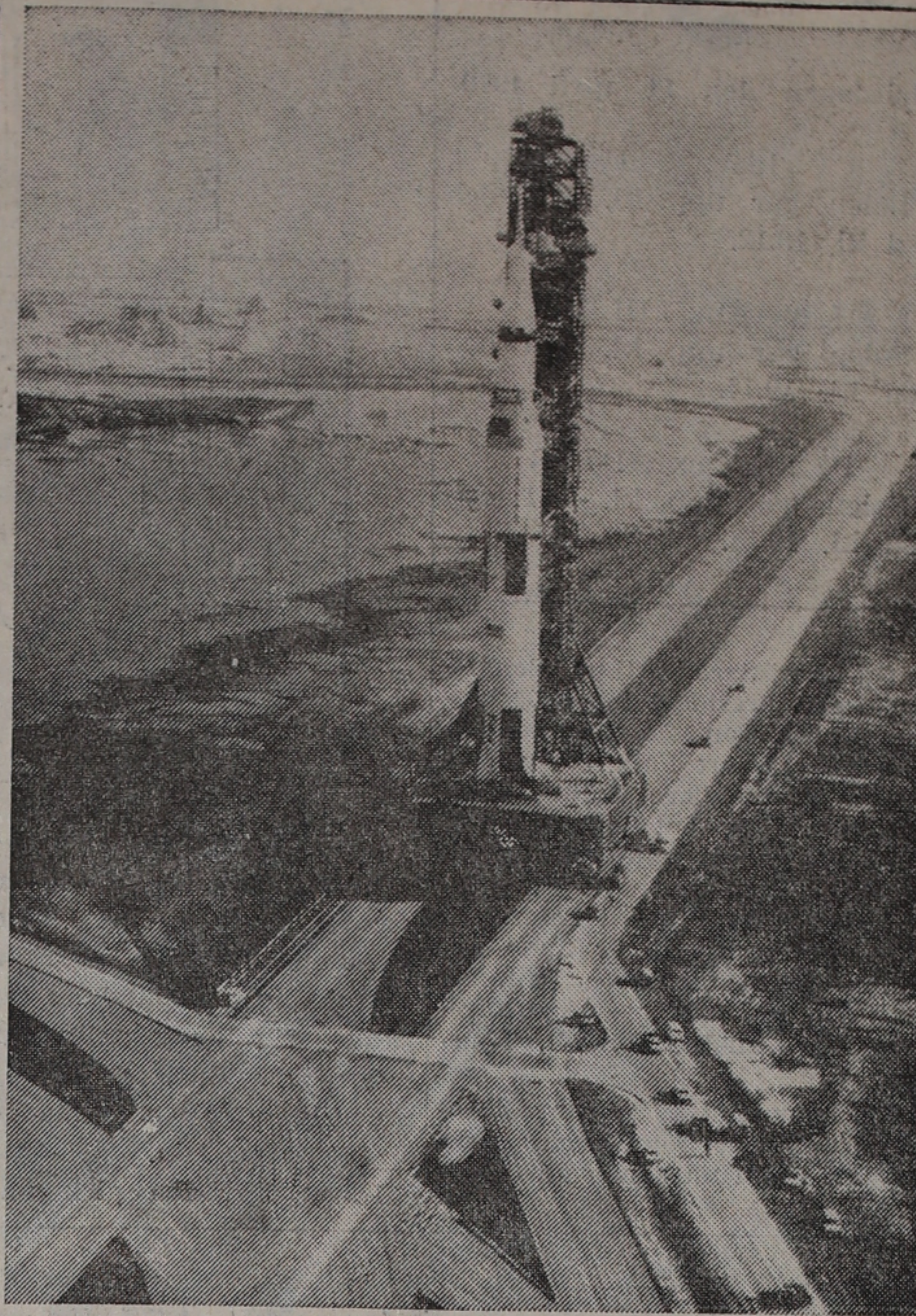
Apollo 13 — tre meter högre än stadshuset i Stockholm — på väg mot startplatta 39 A. Däligt väder kan stoppa uppskjutningen. Det väldiga bandfordonet, på vilket raketen vilar, rullar fram med en hastighet av 1,6 km/timmen.
