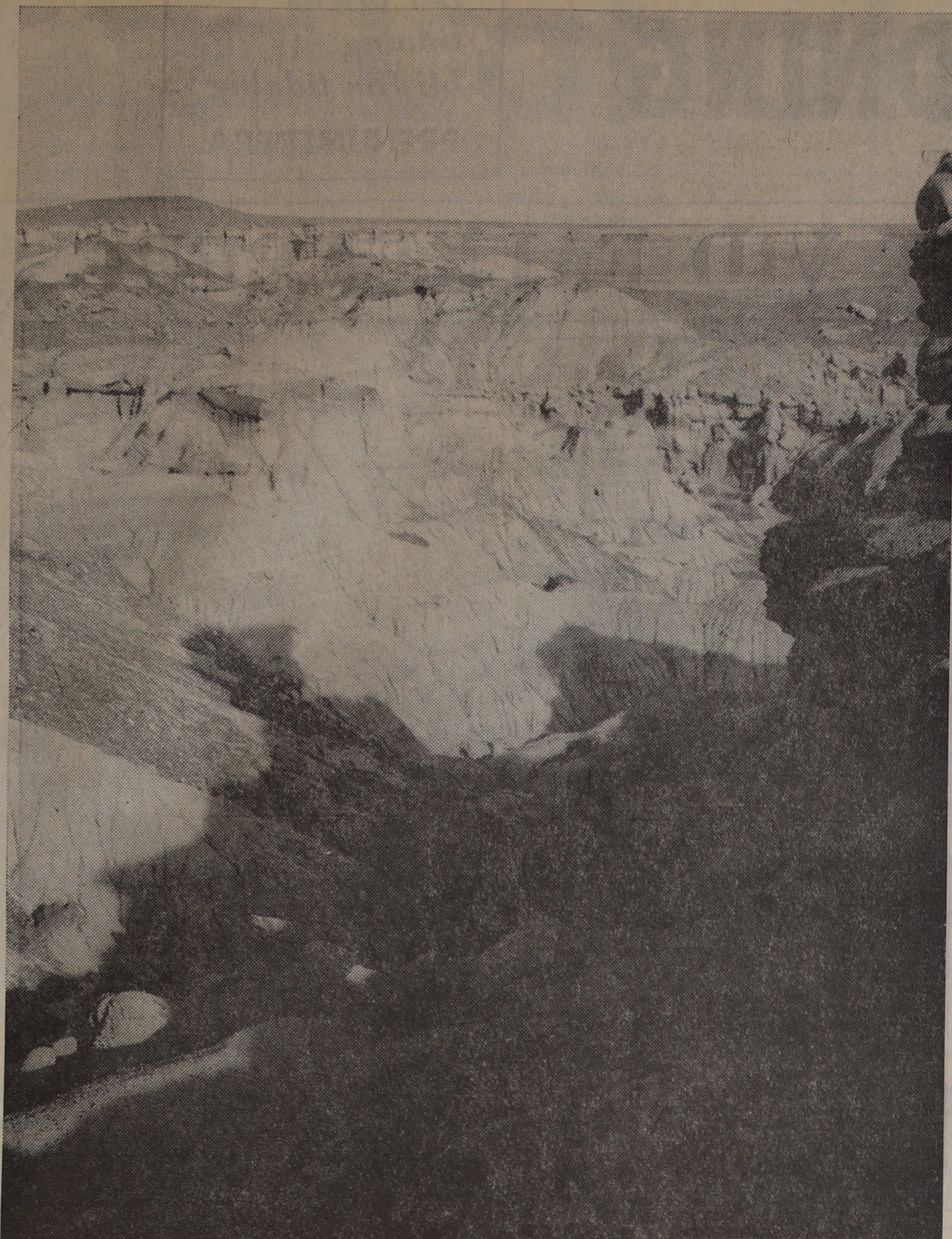
Den vilda floden Colorado grävde sig under 60 miljoner år ner genom de sedimentära bergslagen och skapade fantastiska klippformationer på sin våldsamma färd mot havet — de påminner om katedraler, medeltida riddarborgar, skulptursamlingar, arkader, formerna varierar i det oändliga. Nu är floden reglerad och kvar står dessa underverk som en rapport i sten om naturmaktens spel under miljoner år.
